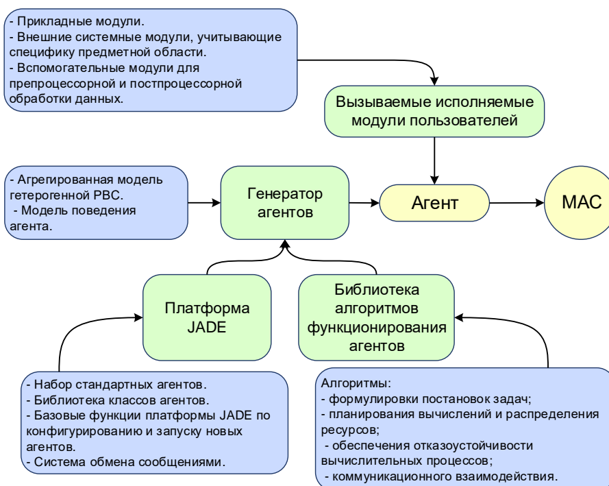
Рисунок 4 – Надстройка к JADE
