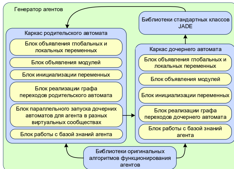
Рисунок 3 – Генерация программного кода агента
