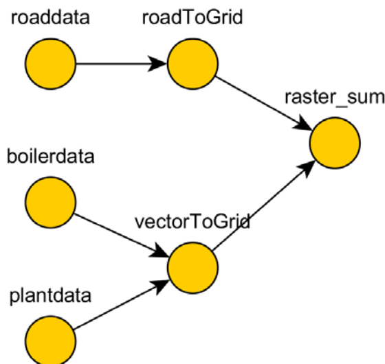
Рис. 1. Полученная семантическая сеть
