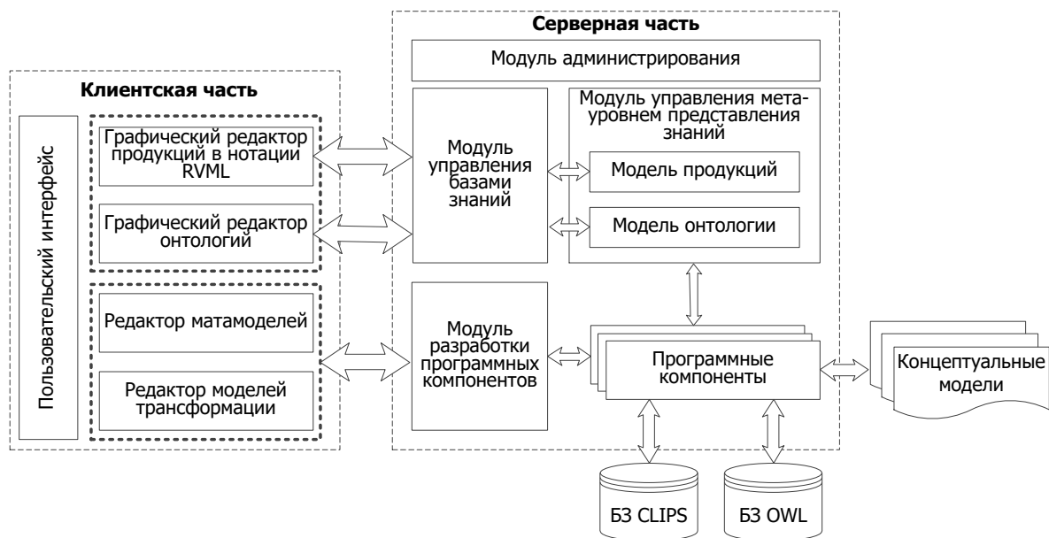
Рисунок 2. Архитектура KBDS
