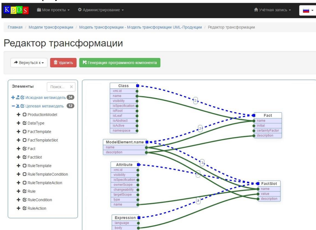
Рисунок 3. Пример экранной формы KBDS: редактор моделей трансформаций (пример фрагмента модели трансформации диаграмм классов UML в модель функций)
